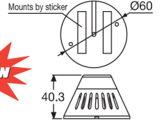
Order No: 2457 Damper Uyarı Sistemi (24V) Damper açık olduğunda ses ve ışık ile uyarı verir. Tipper Warning System (24V) Gives warn by sound and light when the tripper is opened.
